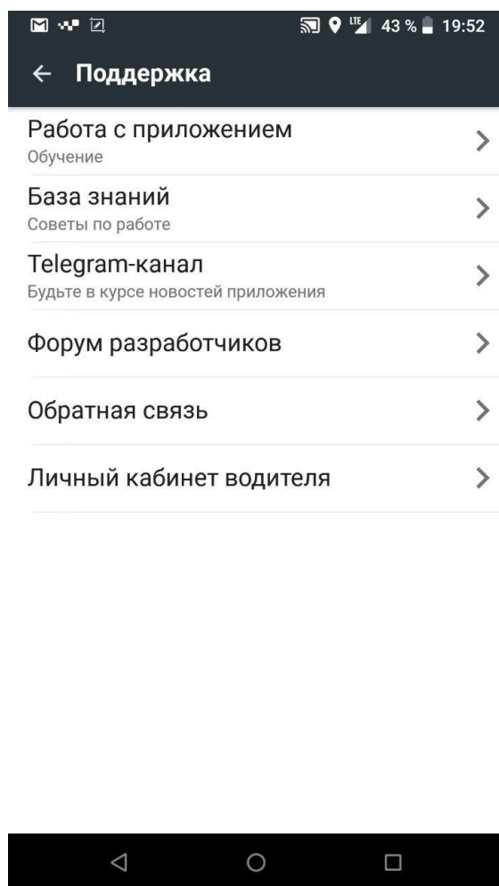
Рисунок 1 – раздел «Поддержка»
